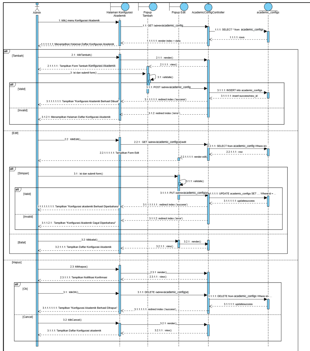
Gambar 3. 33 Sequence Diagram Mengelola Konfigurasi Akademik
