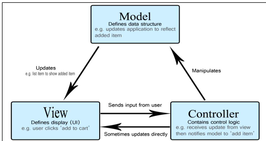
Gambar 2. 3 Arsitektur Model-View-Controller
