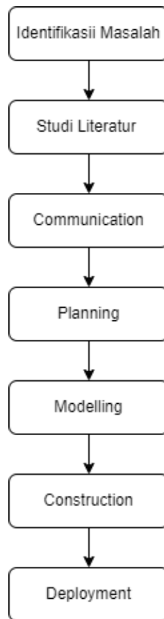
Gambar 3. 1 Tahapan Penelitian
